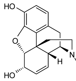
Morphine Verlag Helvetica Chimica Acta
